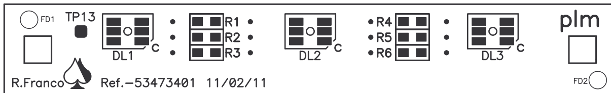
Serigrafía de Componentes
